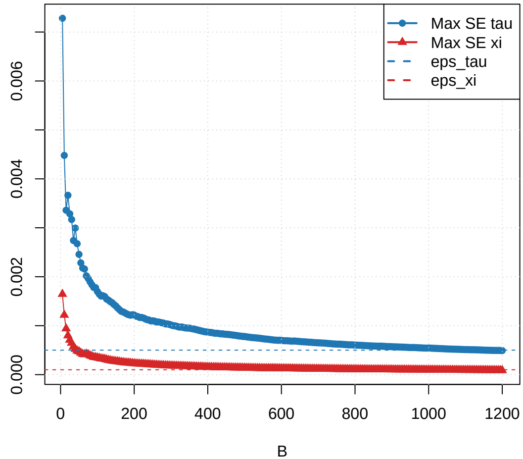
Max SE
