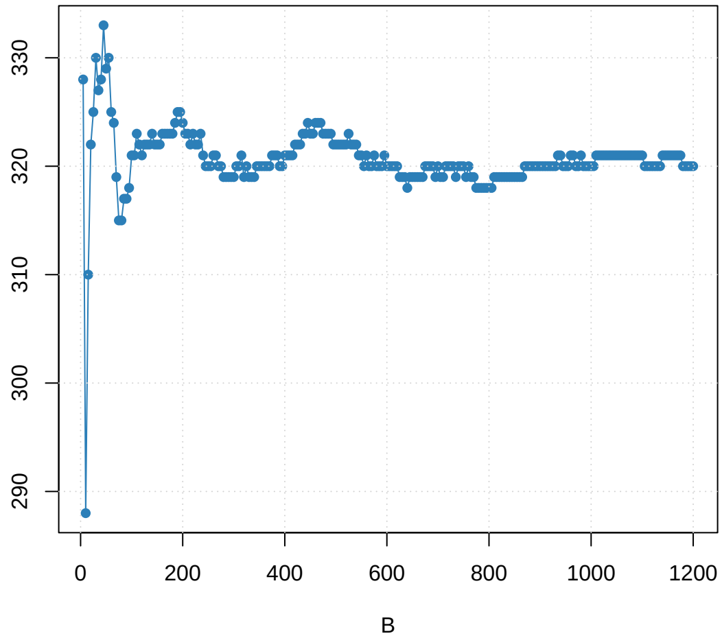
Max SE
